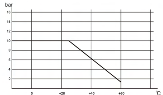
温度 - 压力表
