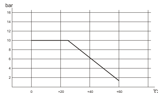
温度 - 压力表
