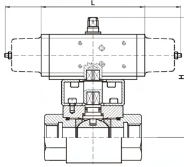
单气动弹簧复位型
