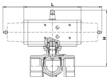
单气动弹簧复位型
