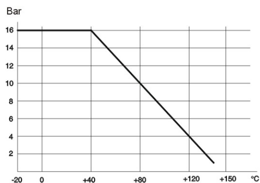
温度 - 压力表
