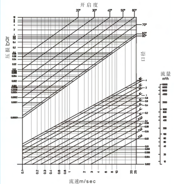
流量 / 压力图-压损及 Kv值
